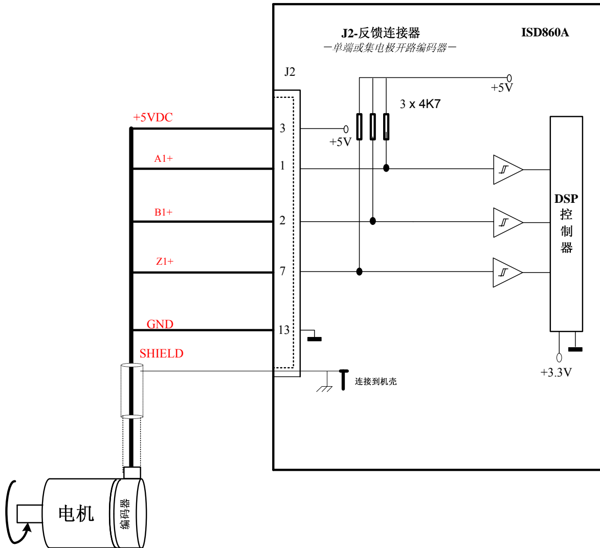
图 3.8. J2 – 单端/或集电极开路编码器连接
