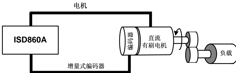
图 2.4. 有刷直流旋转电机，位置/速度/转矩控制，电机上带增量编码器
