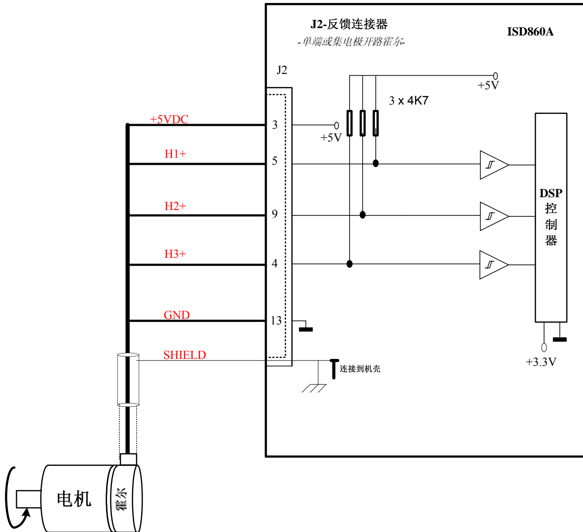
图3.10. J2 -单端或/集电极开路霍尔连接
