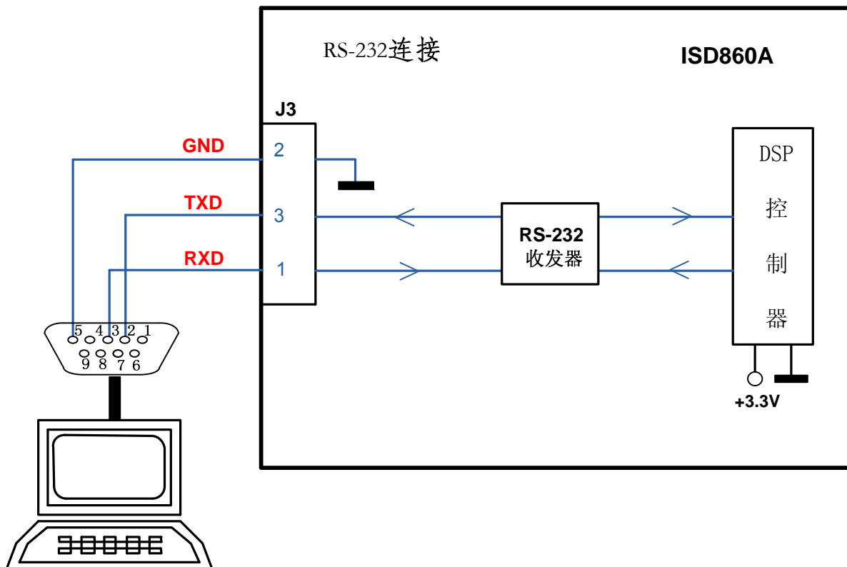
图 3.14. J3—串行 RS-232 连接
