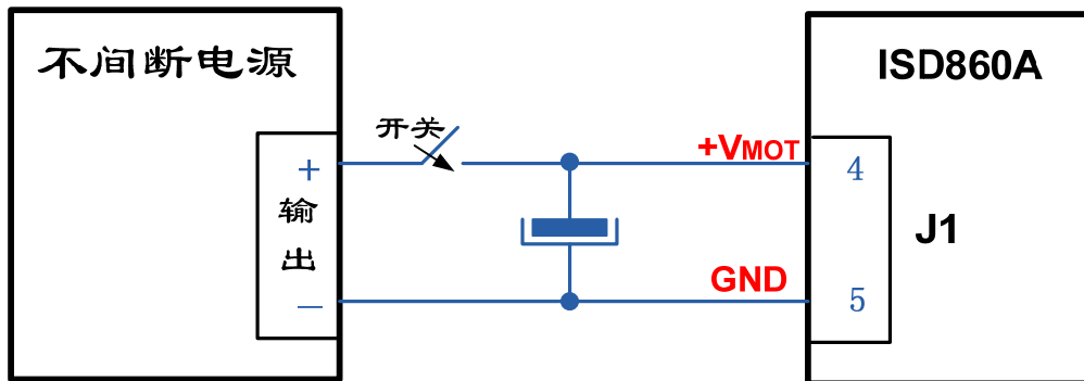
图 3.7. J8—电机电源连接—另一种冲击电流限制
