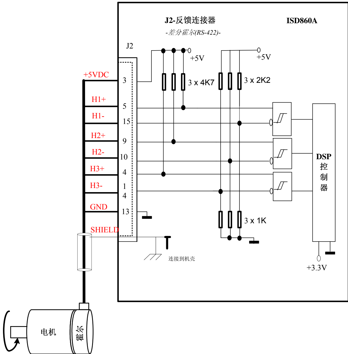
图 3.11. J2 - 差分(RS-422)霍尔连接
