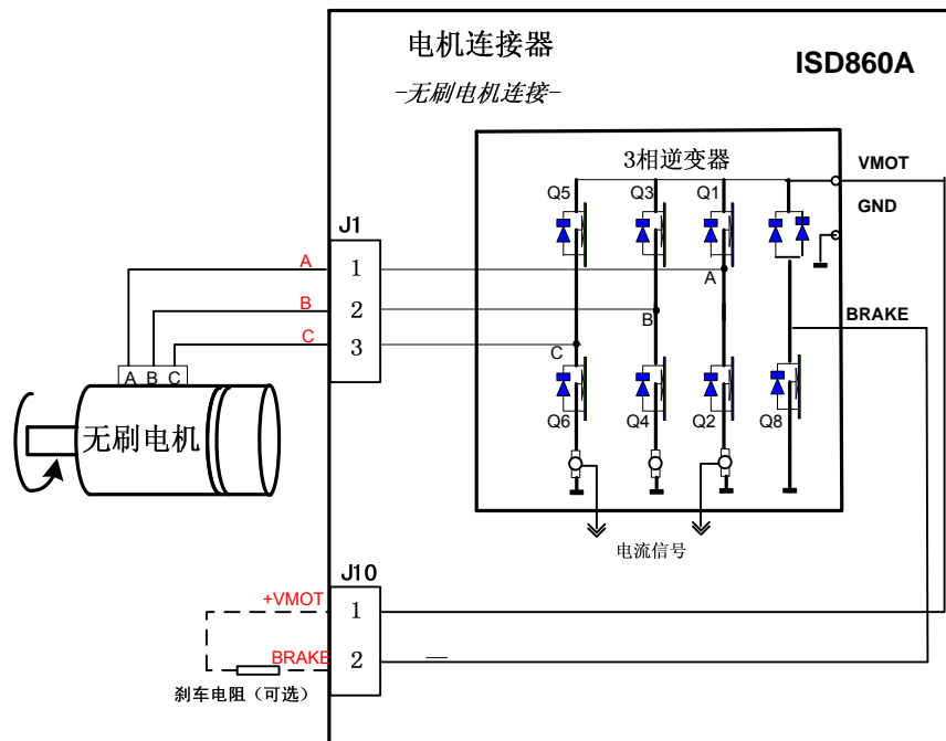
图 3.4. J1—无刷电机连接
