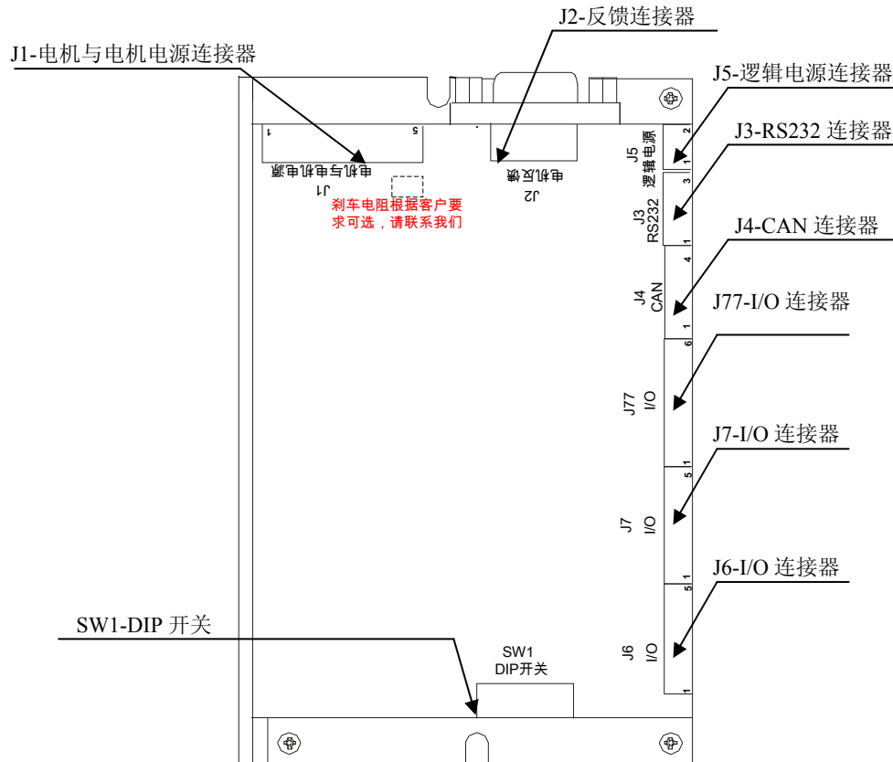
图 3.2. ISD860A 驱动器连接器布局
