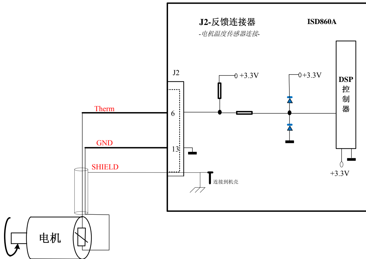
图 3.12. J2 - 电机温度传感器连接
