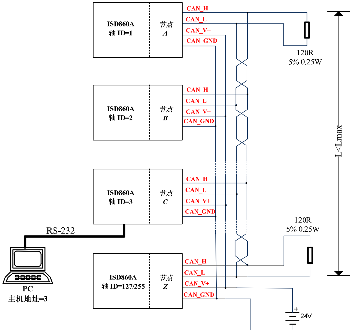
图 3.16. 多轴 CAN 网络
