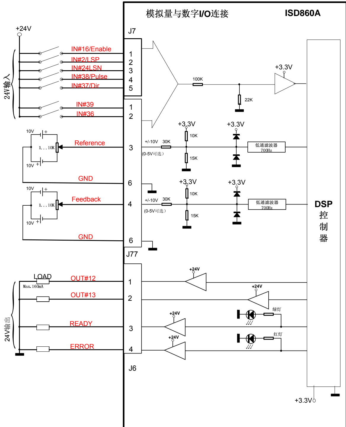
图 3.13. 一模拟量与数字 I/O 连接
