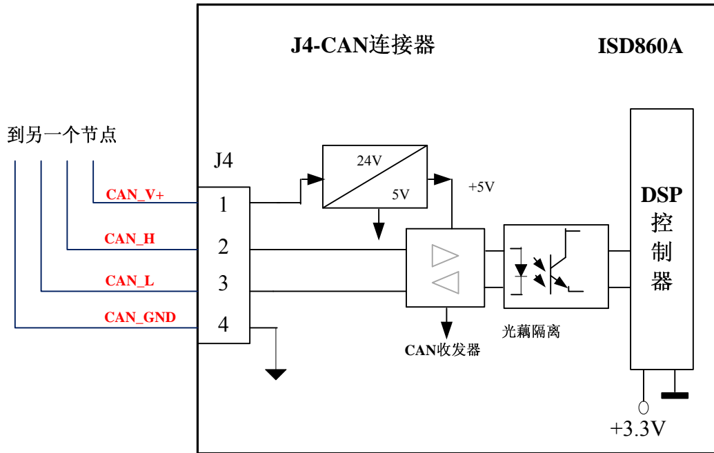
图 3.15. J4-CAN 连接器
