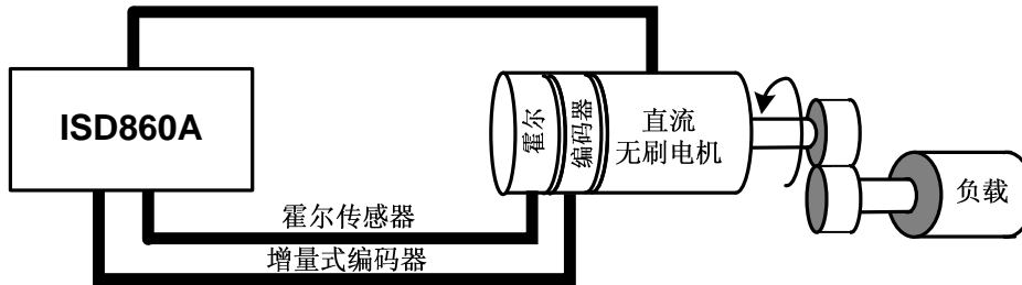
图 2.3. 直流无刷旋转伺服电机，位置/速度/转矩控制，电机上带霍尔传感器与增量编码器
