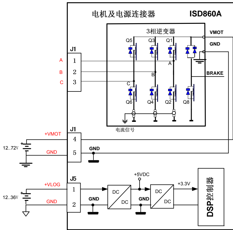
图 3.3. 电机和电源连接
