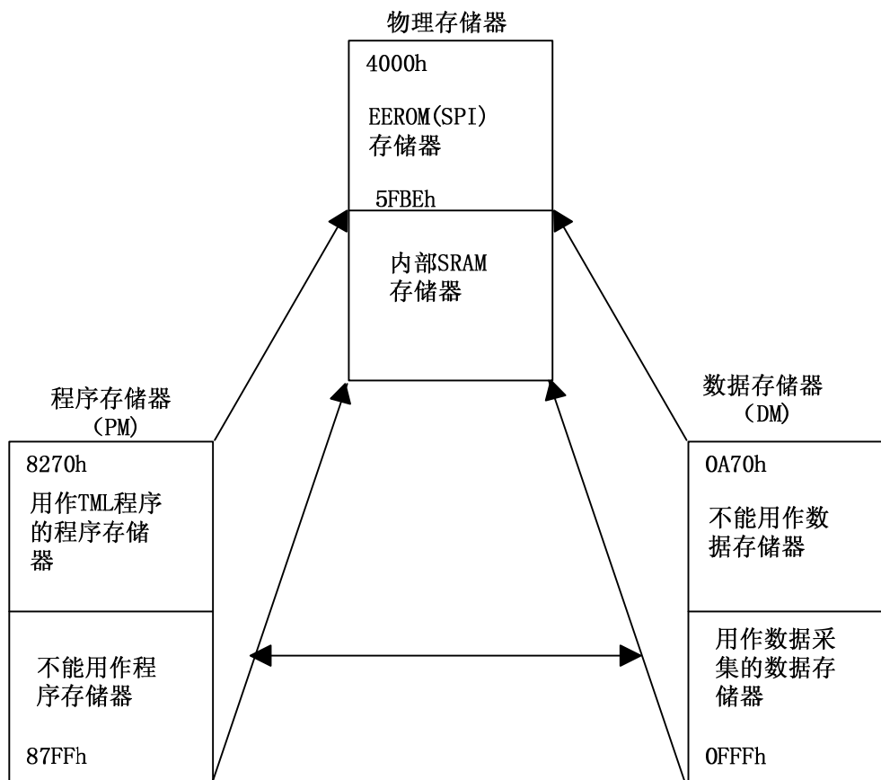
图 7.1. ISD860A / ISD860A-RS232/CAN 存储器映射
