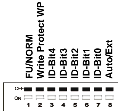
图 3.17 SW1-DIP 开关为执行 CAN 通信
