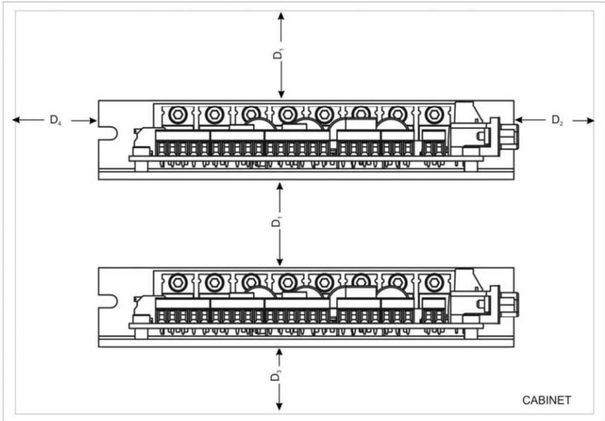
图 3.1. ISD860A 放在机箱中安装推荐
