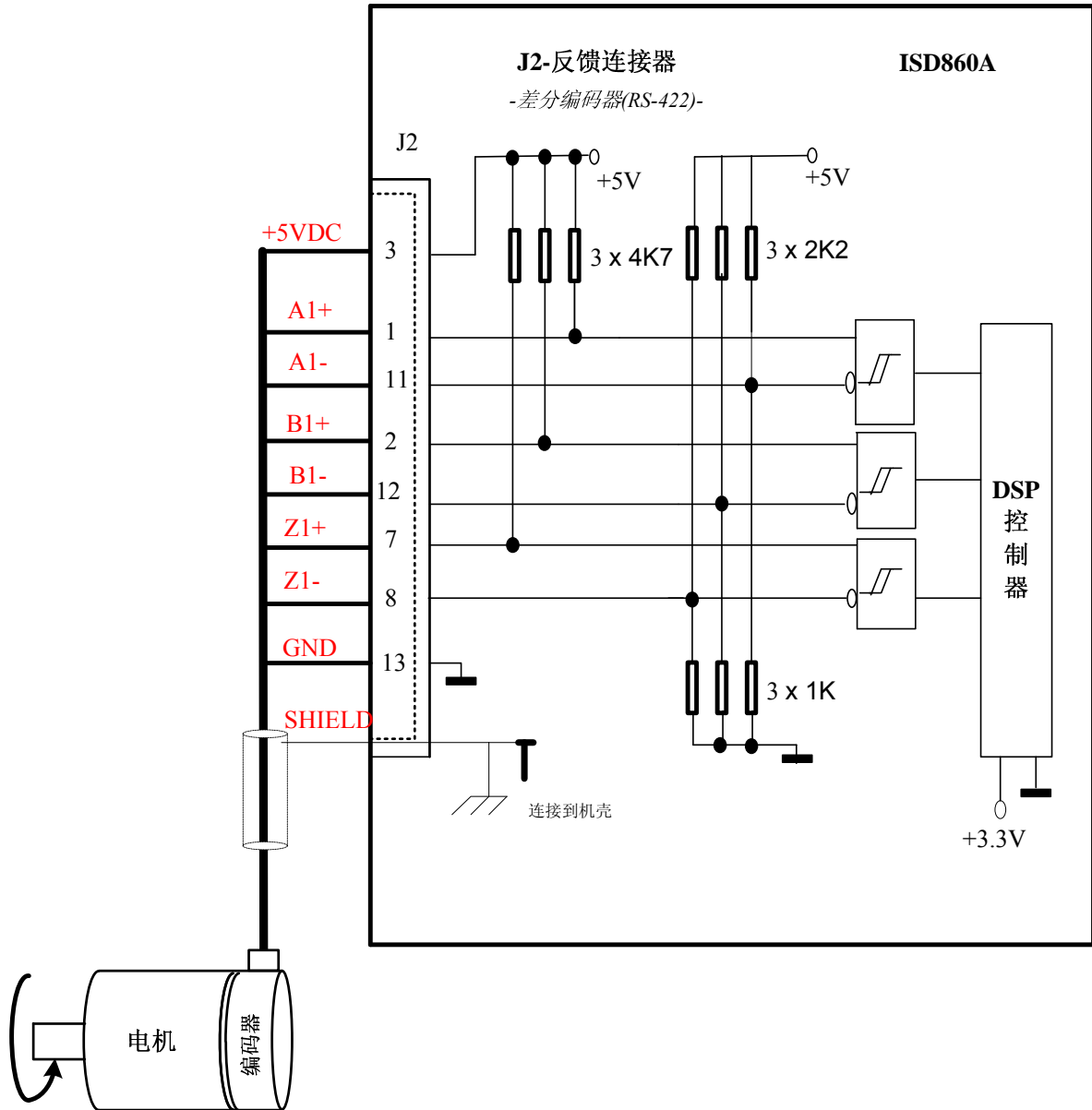
图 3.9. J2 –差分 (RS-422) 编码器连接
