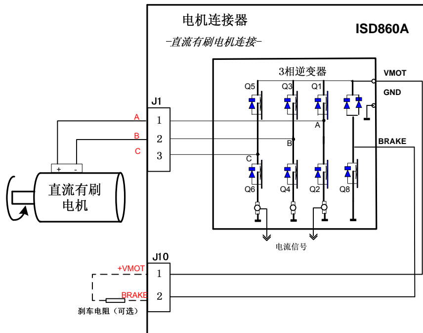
图 3.5. J1—直流有刷电机连接
