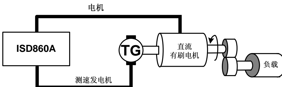
图 2.5. 直流有刷旋转伺服电机，速度/转矩控制，电机带测速发电机
