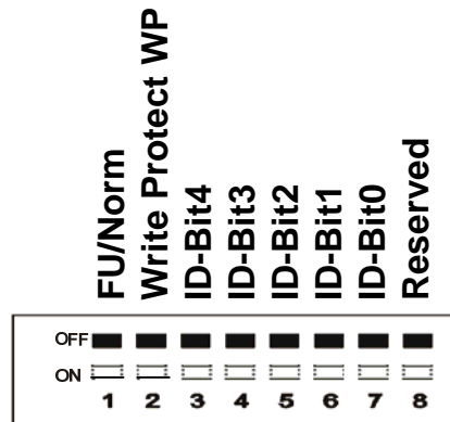
图 3.18 SW1-DIP 开关为执行 CANopen 通信
