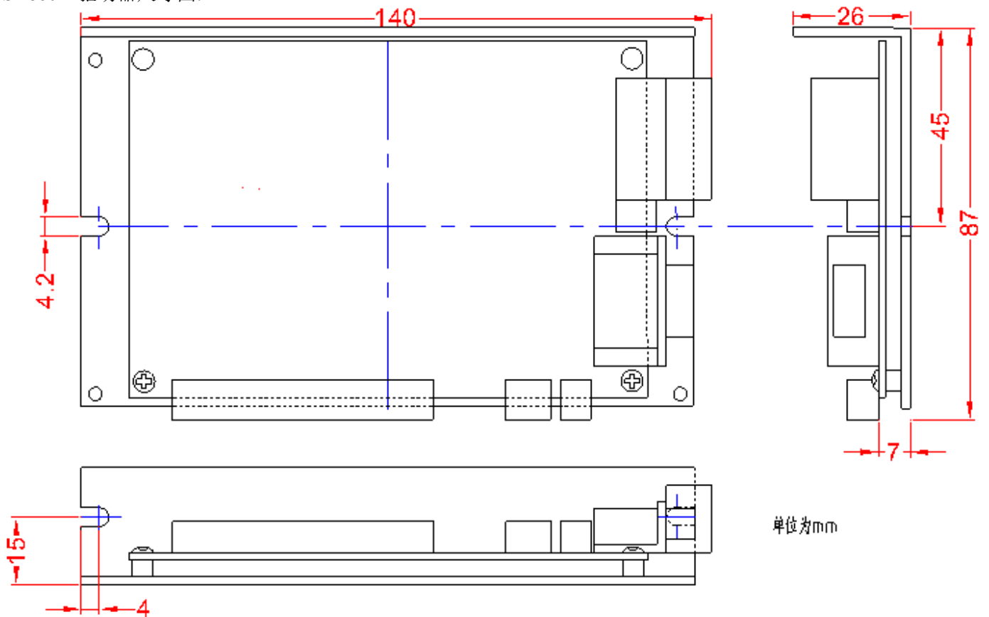
图 2.7. ISD860A 驱动器尺寸图
