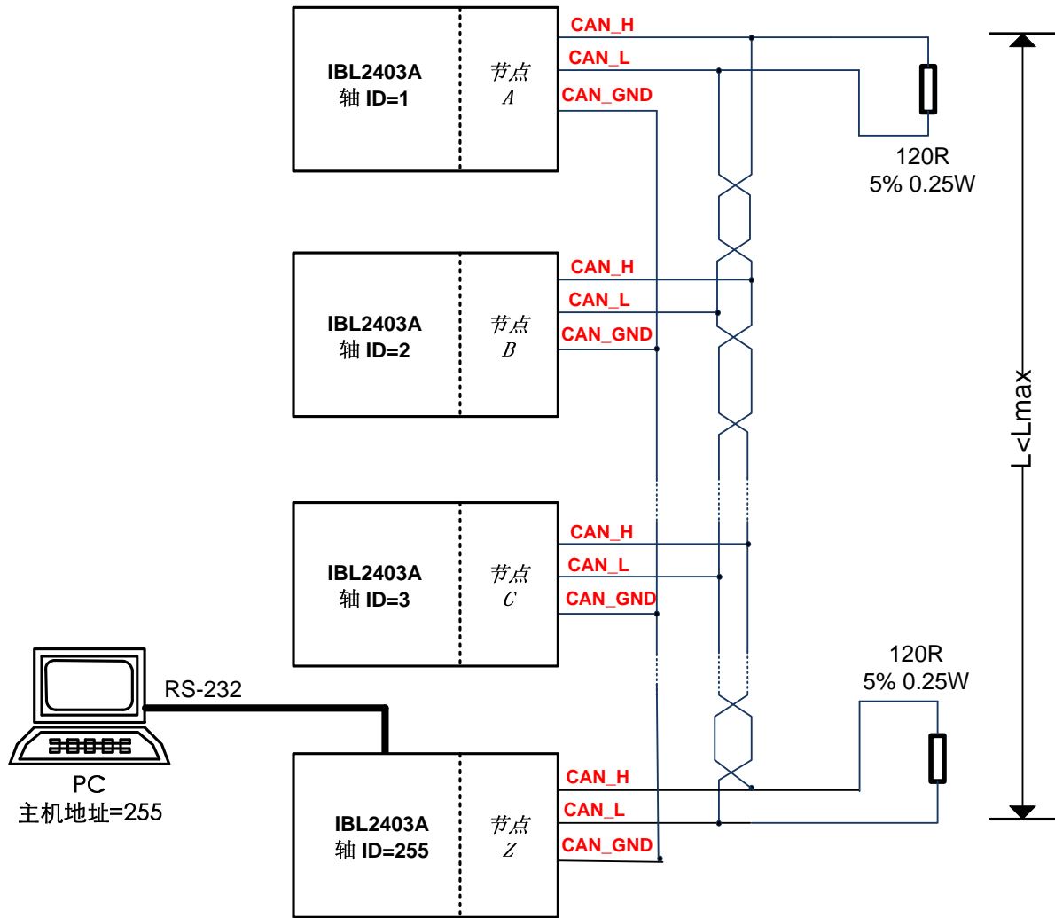
图 3.19. 多轴 CAN 网络
