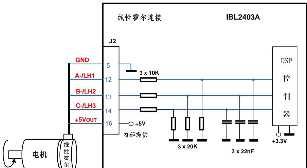
图 3.14. 线性霍尔连接
