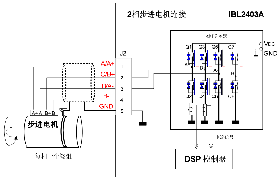
图 3.7. 步进电机连接
