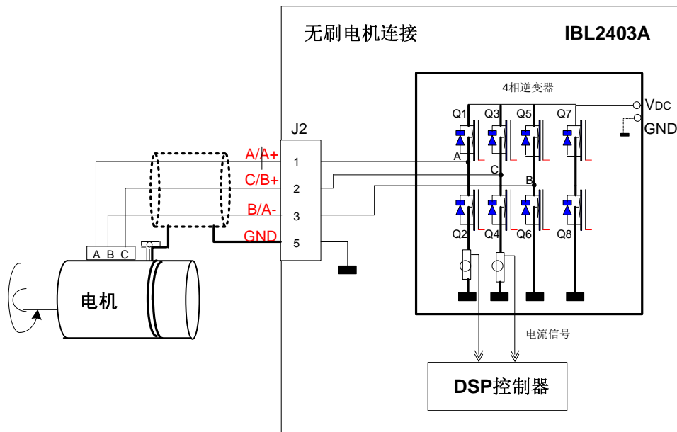
图 3.6. 无刷电机连接
