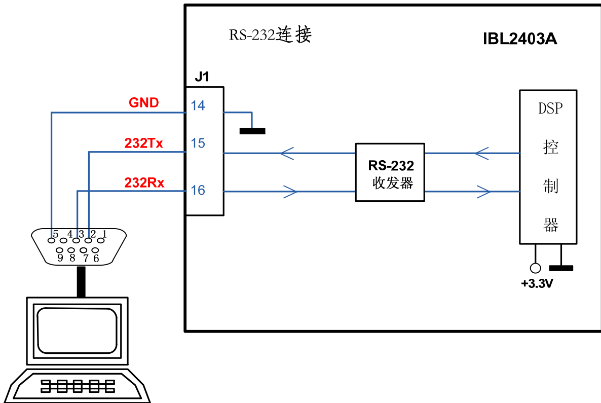
图3.17. 串行RS-232 连接
