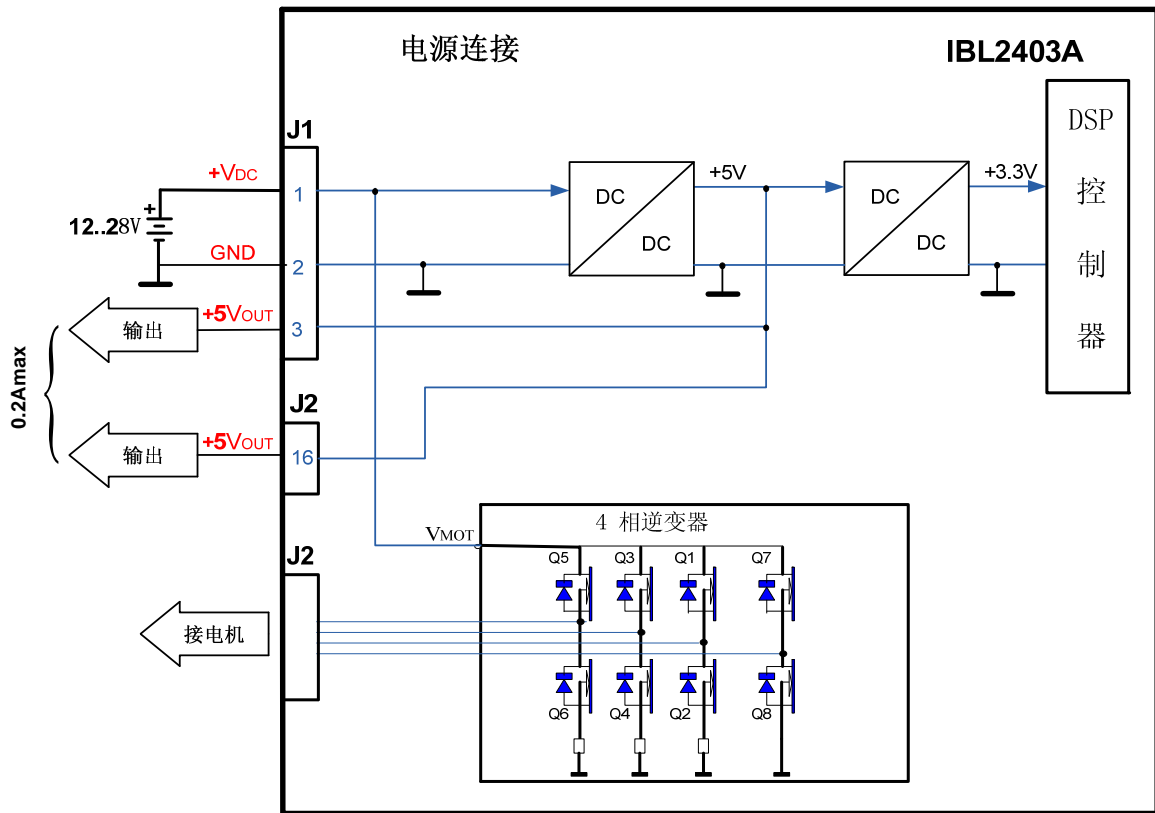
图 3.16. 电源连接
