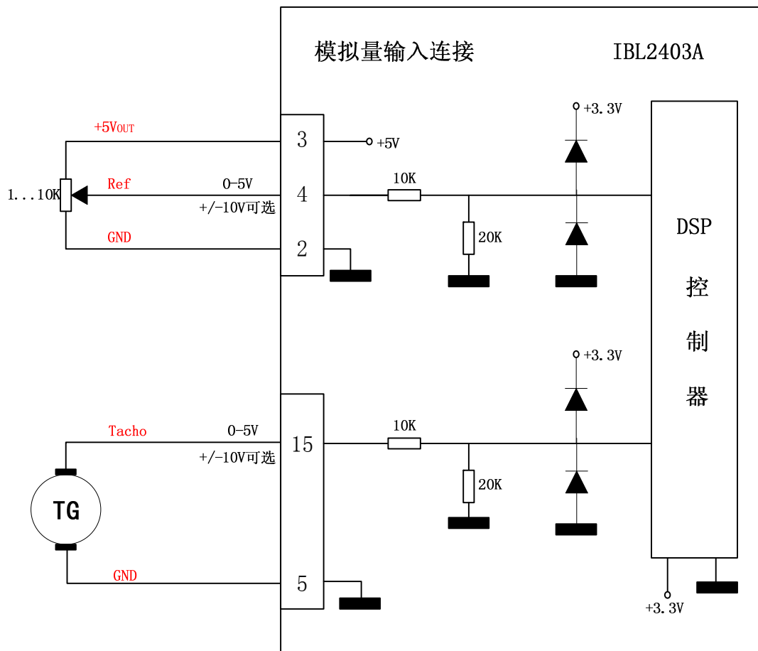
图 3.5. 模拟量输入连接
