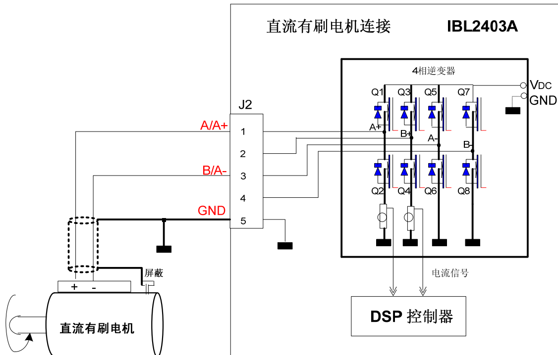
图 3.10. 直流有刷电机连接
