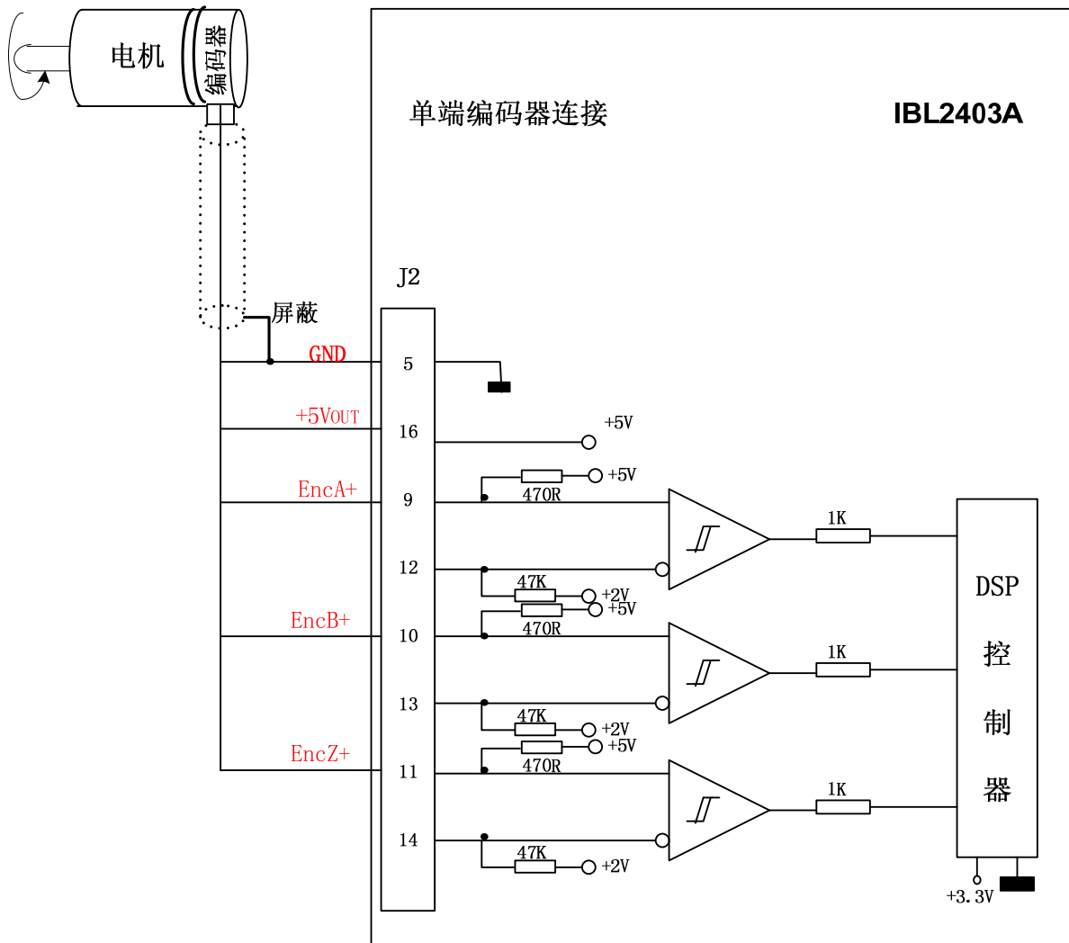
图 3.11. 单端编码器连接
