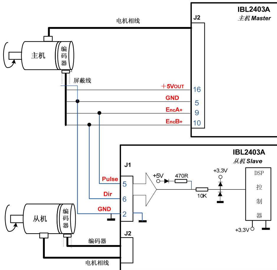
图 3.21. 主从编码器连接—通过脉冲+方向接口输入
