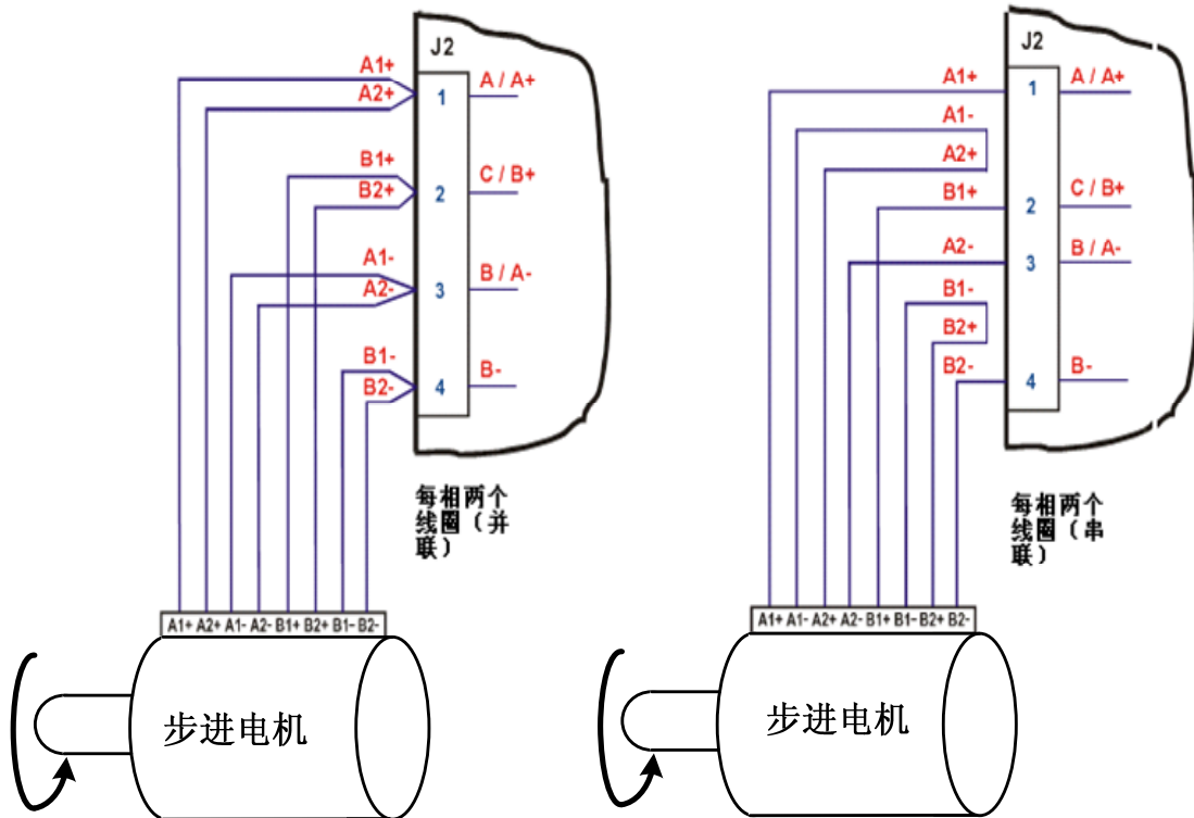
图 3.8. 步进电机连接
