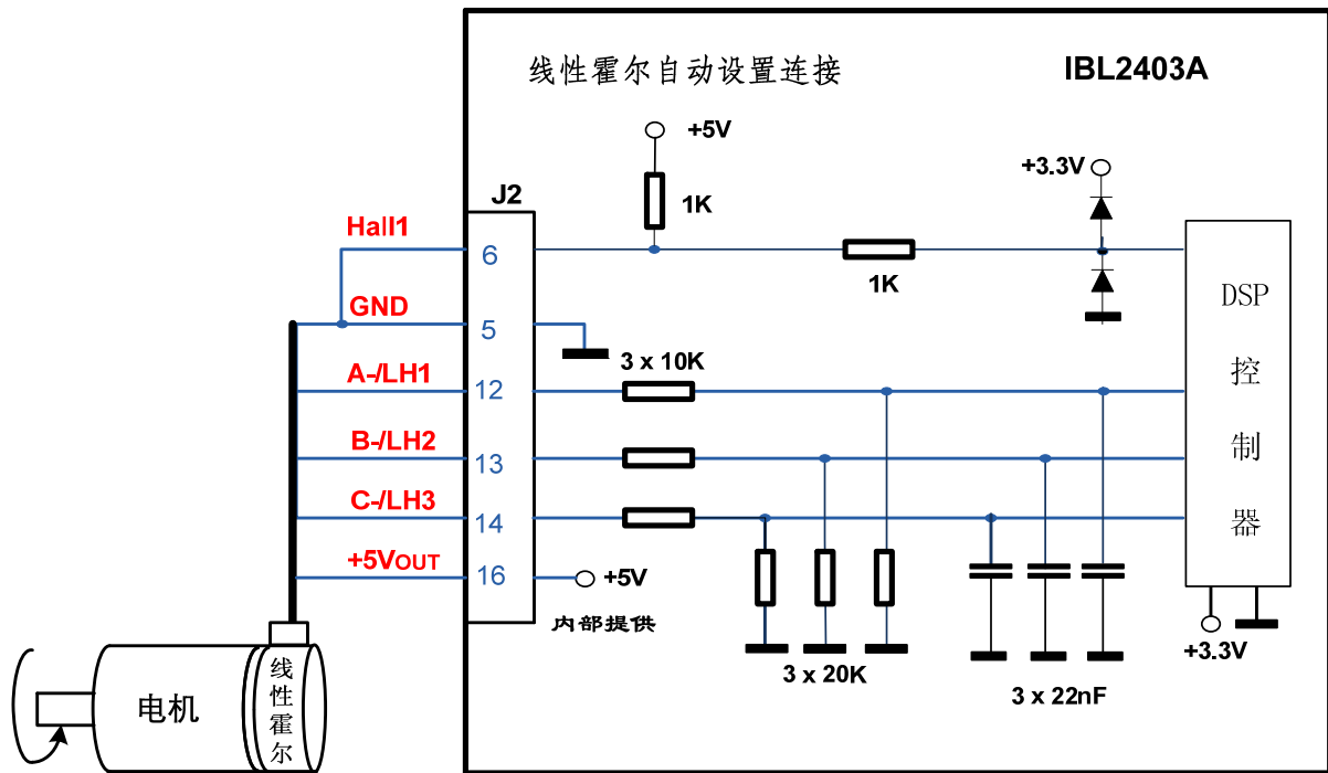
图 3.15. 线性霍尔自动设置连接
