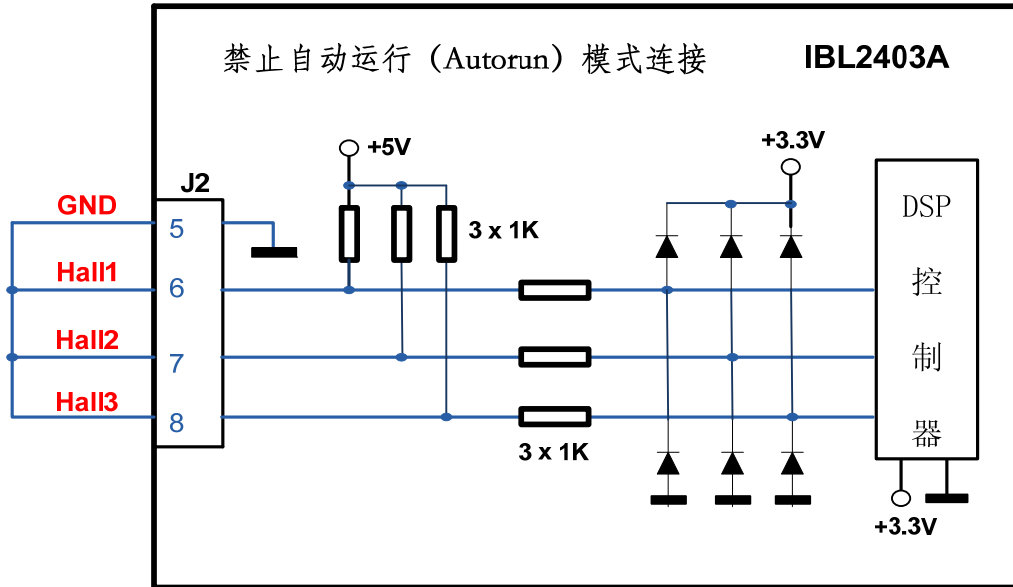
图 3.20. 禁止自动运行 (Autorun) 模式连接
