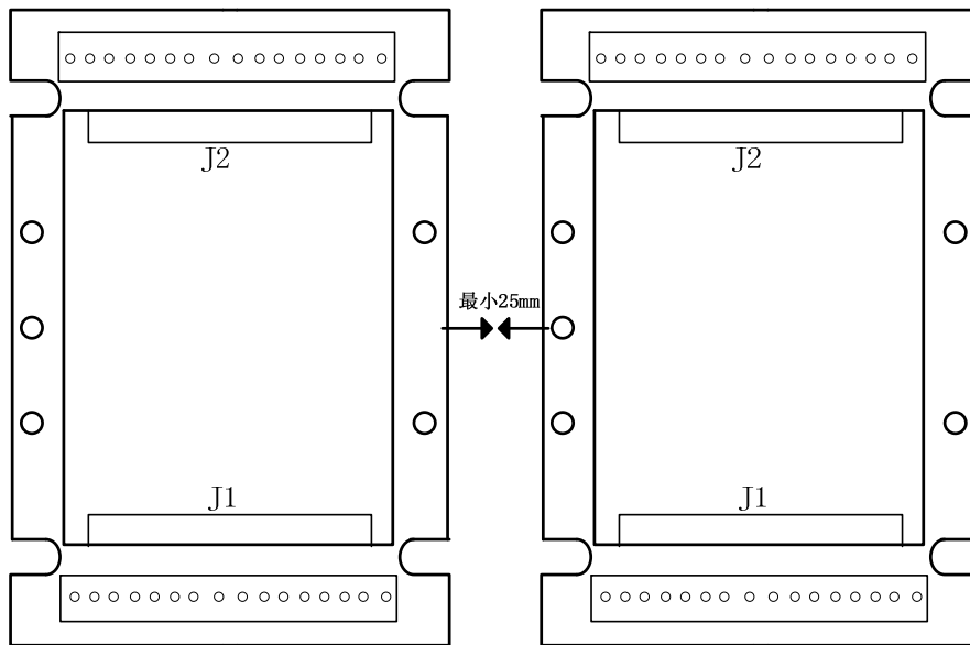
图 3.1. IBL2403A 驱动器安装
