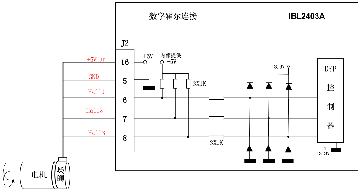
图 3.13. 数字霍尔连接
