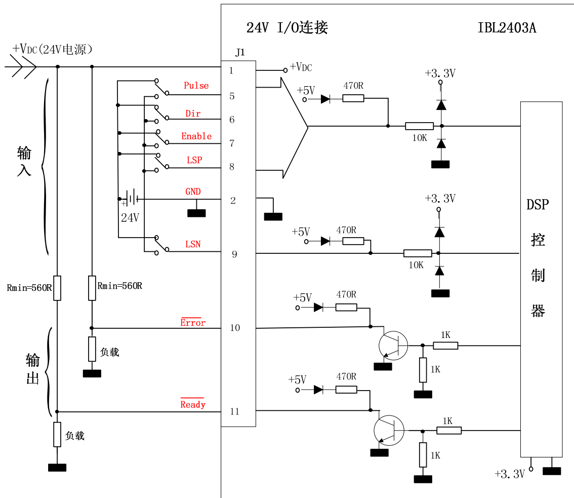
图 3.3. 24V 数字 I/O 连接
