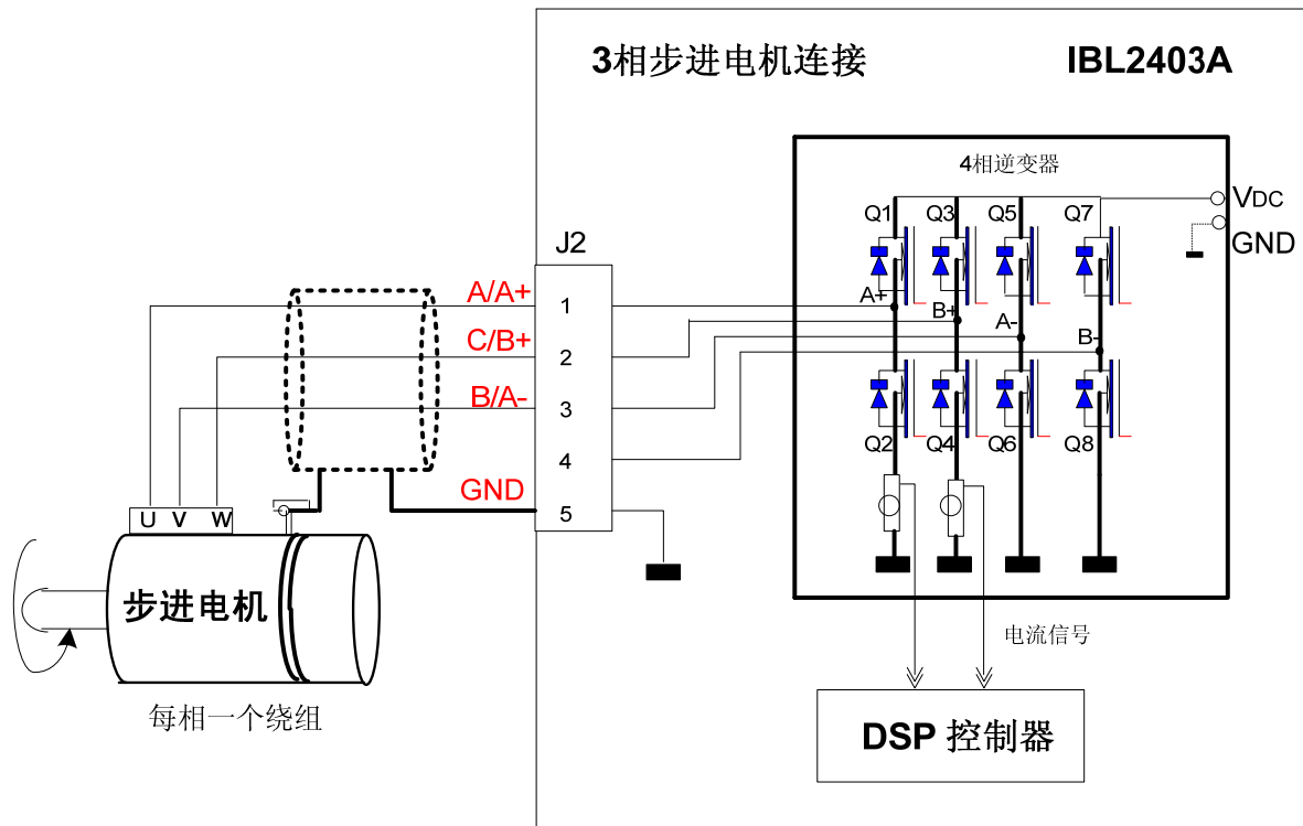
图 3.9. 3 相步进电机连接
