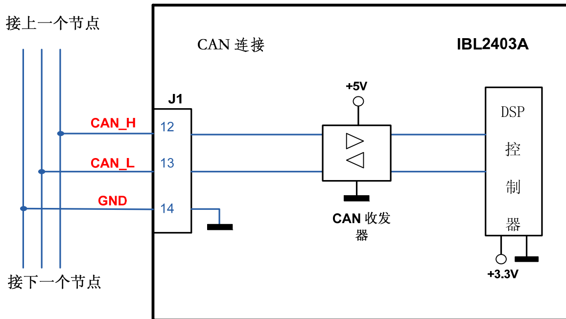
图3.18. CAN 连接
