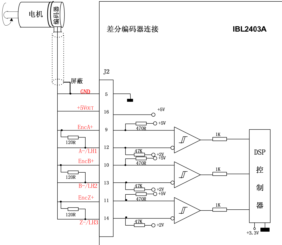
图 3.12. 差分编码器连接
