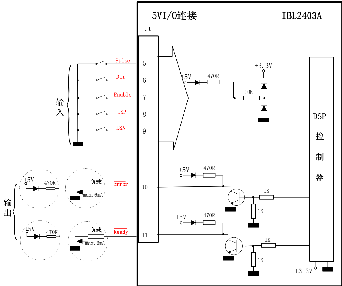
图 3.4. 5V 数字 I/O 连接
