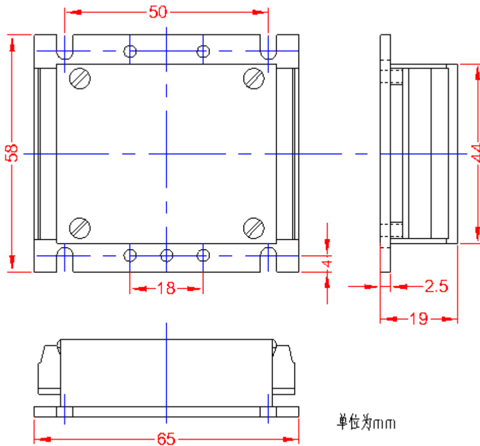
图2.11. IBL2403A 驱动器尺寸图
